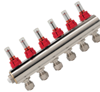
► Debili Kontrollü Kollektör 1" 16x2 (PN 10)
